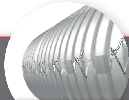
Gancho serpiente bastón para las alcantarillas de Ø1.05 a Ø1.83 m
